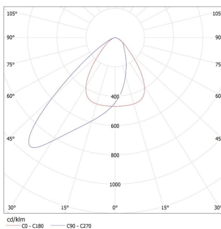
KANLUX S.A. (kat 33474) FL AGOR/A LED 150W NW / LDC (Polar)
